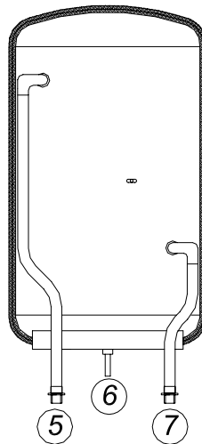
CT210/20 bakifrån
