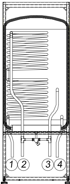
CT210/20 Framifrån
